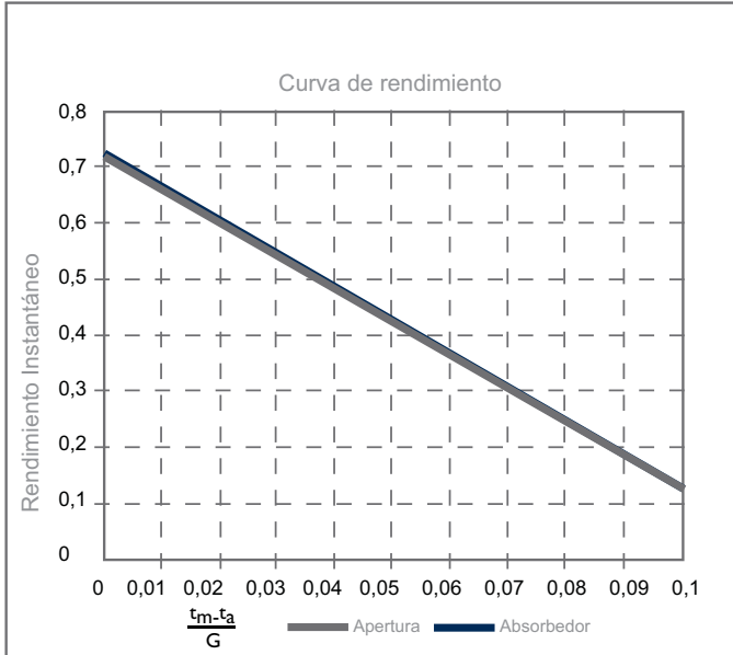
Curva de rendimiento captador Eurener 2.5
