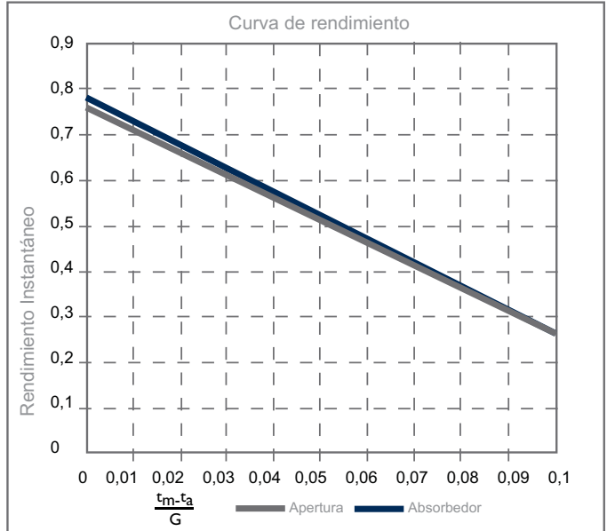
Curva de rendimiento captador Eurener 2.5 Selectivo
